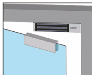
Montaż z uchwytem BK-350UL
