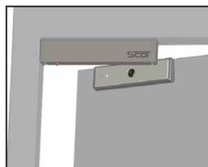
Montaż standardowy / z uchwytem BK-350I
