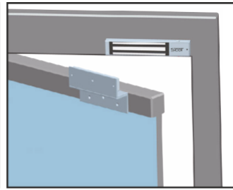
Montaż z uchwytem BK-1500ZL2
