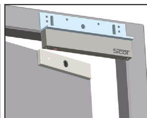
Montaż z uchwytem BK-800L2, BK-800LC2
