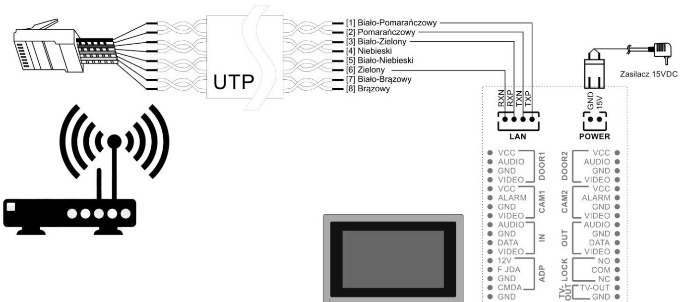
Rys. Połączenie wg standardu EIA 568B
